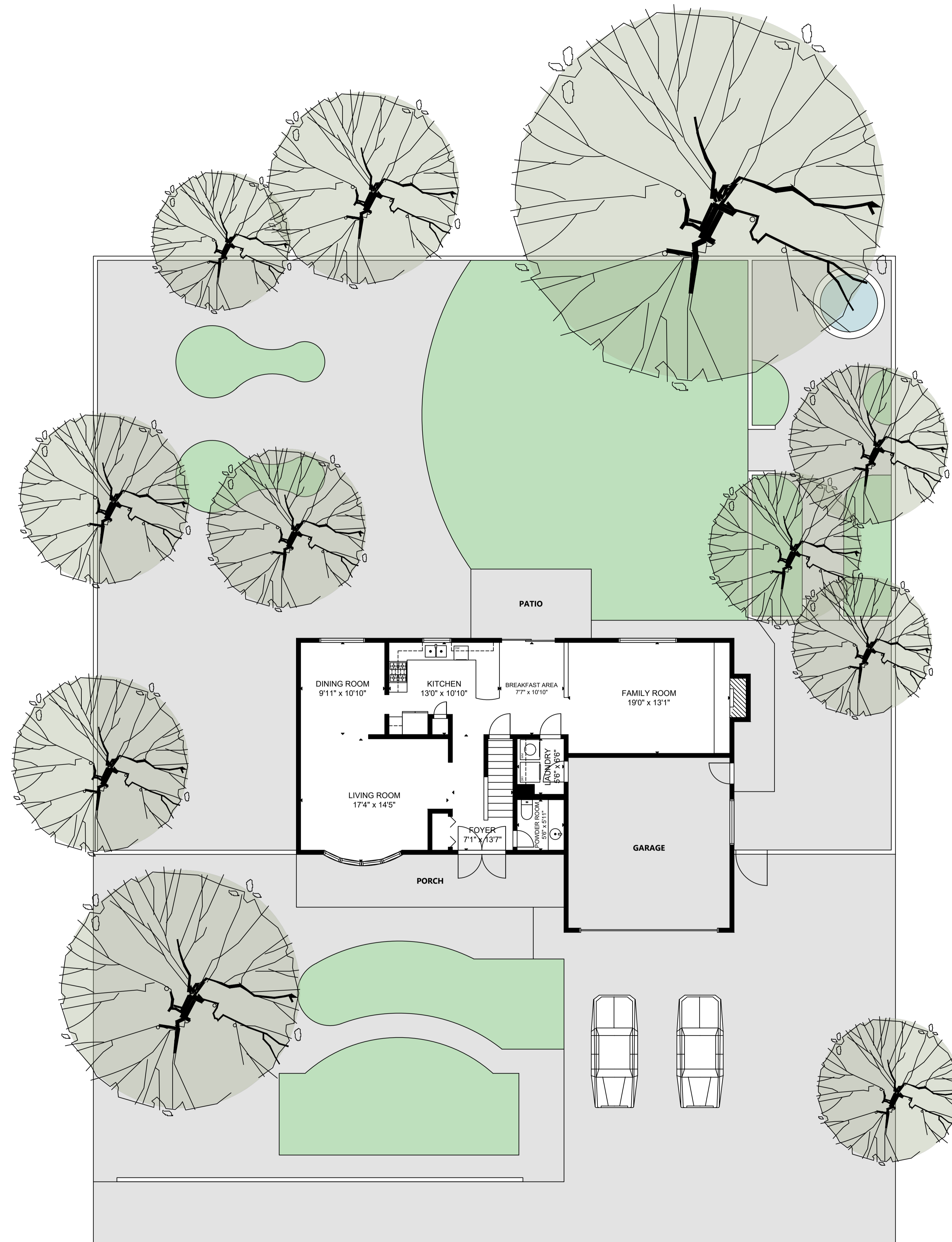
SITEPLAN
