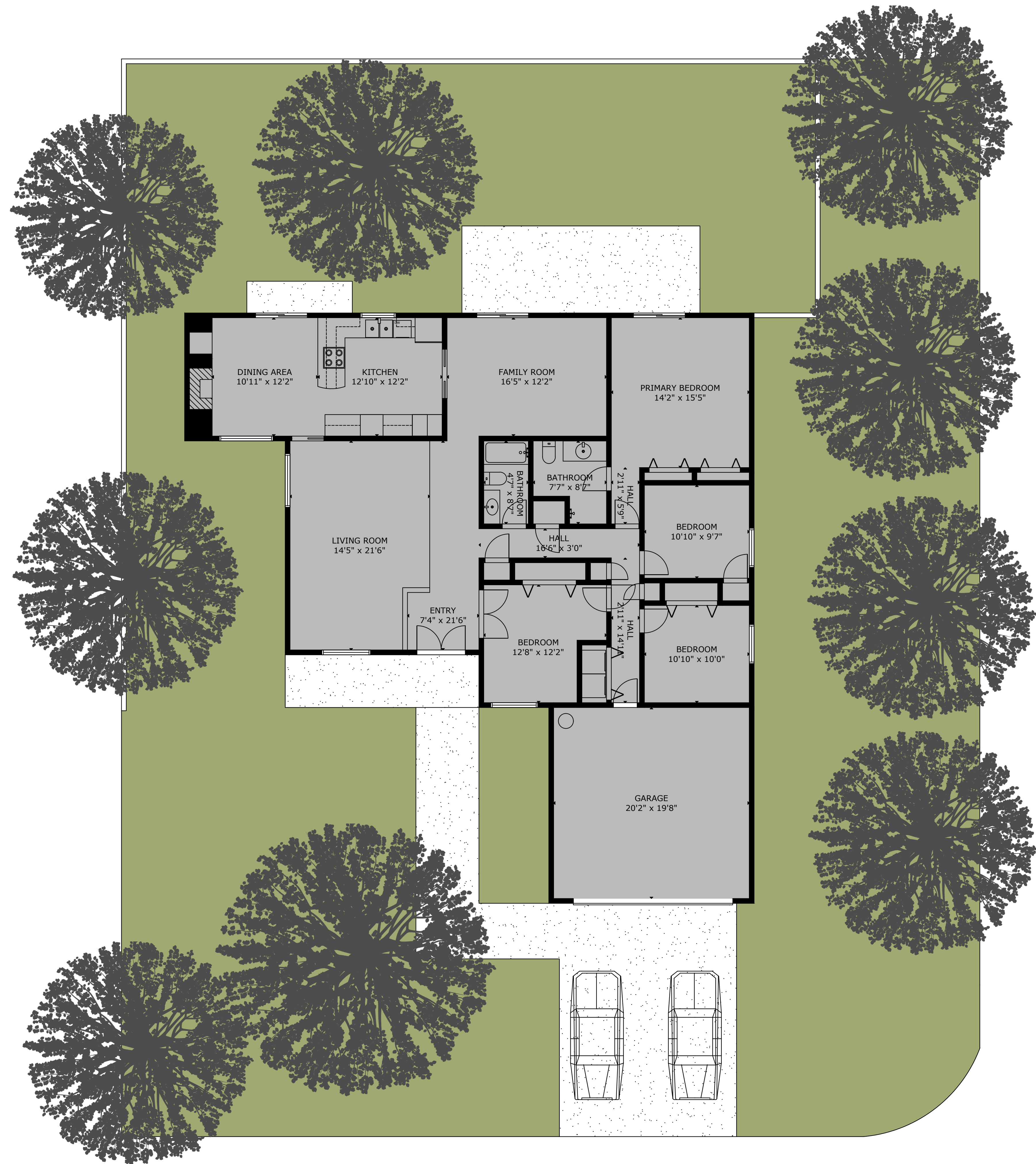
SITEPLAN
