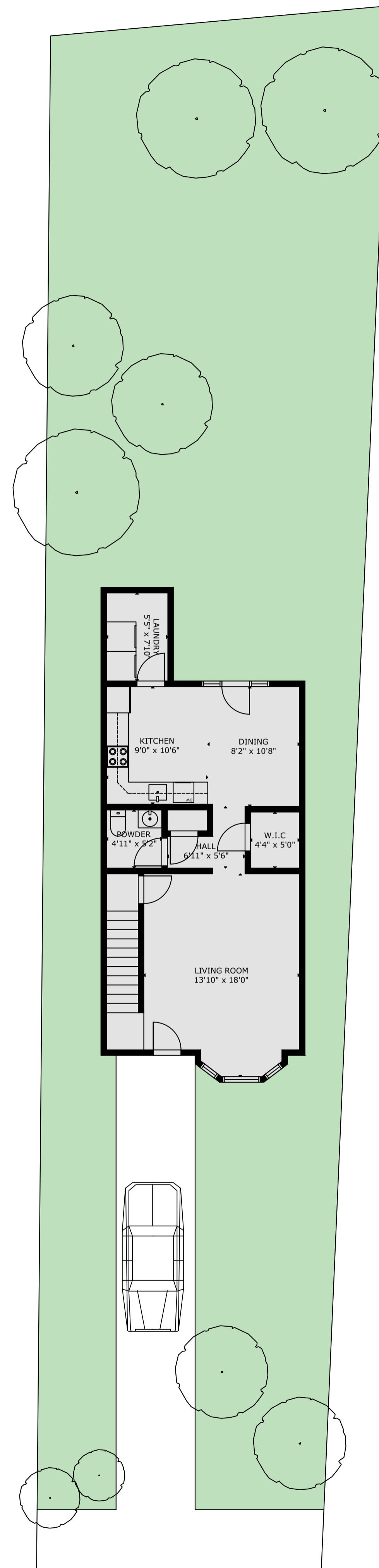
SITEPLAN
