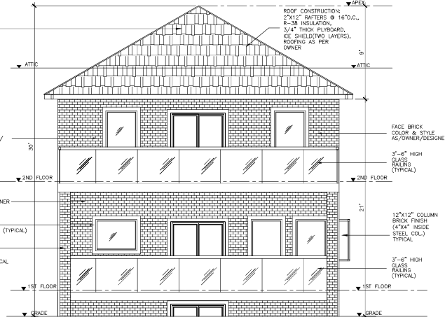
REAR ELEVATION SCALE: 1/4"=1'0"
