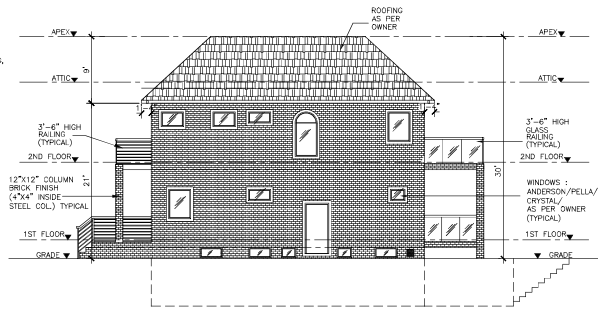
RIGHT SIDE ELEVATION SCALE: 1/8"=1'0"
