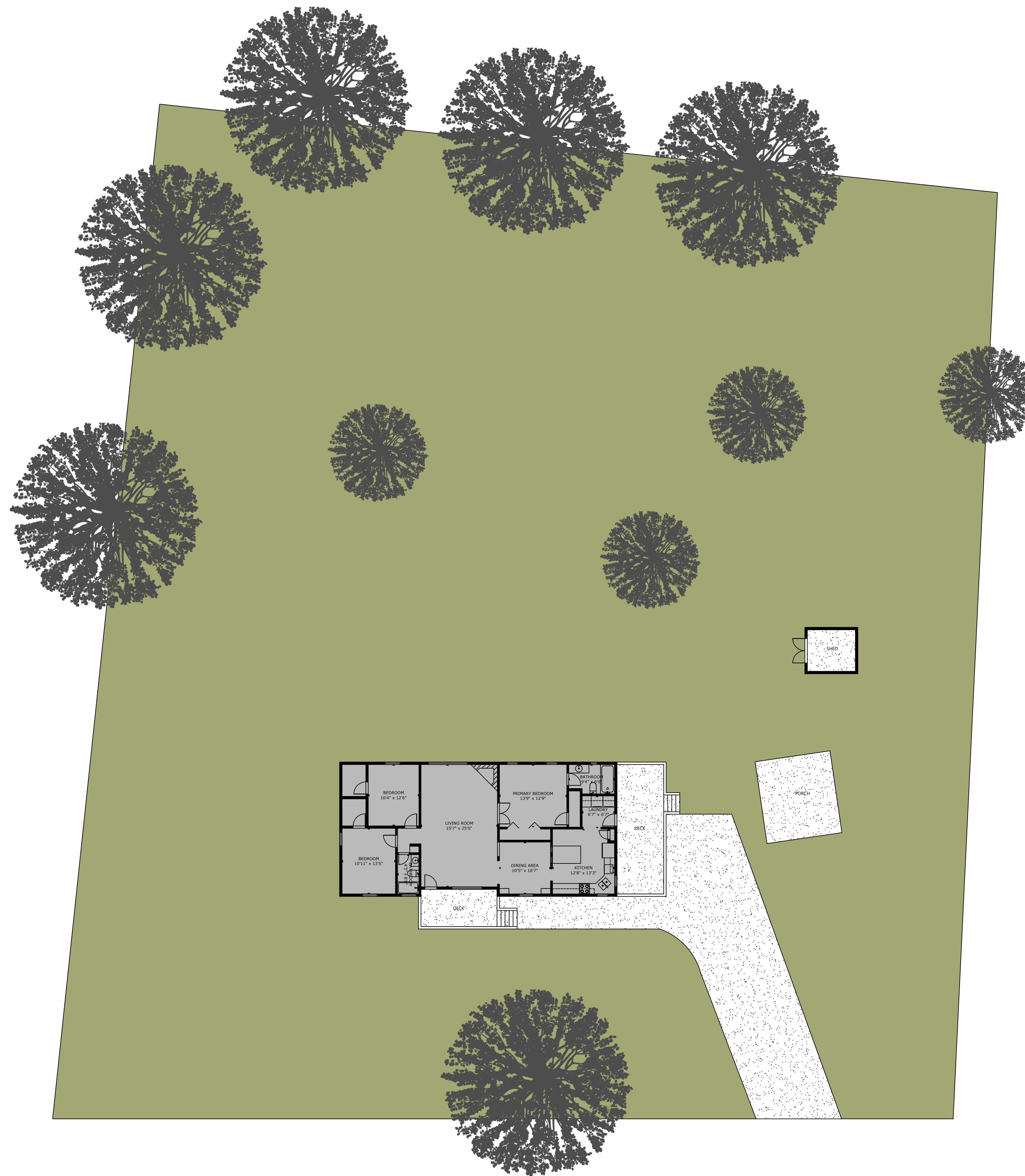
SITEPLAN
