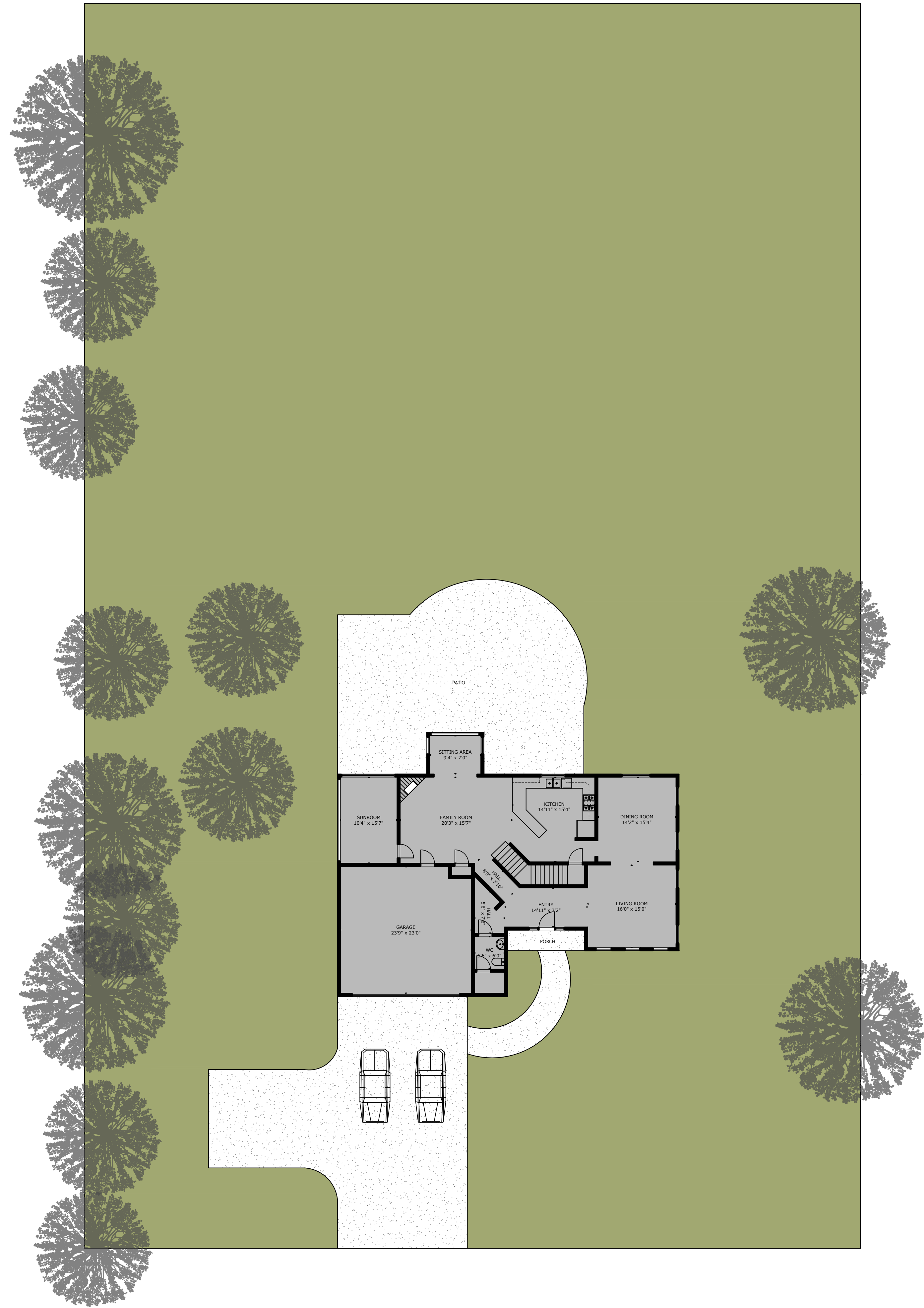
SITEPLAN
