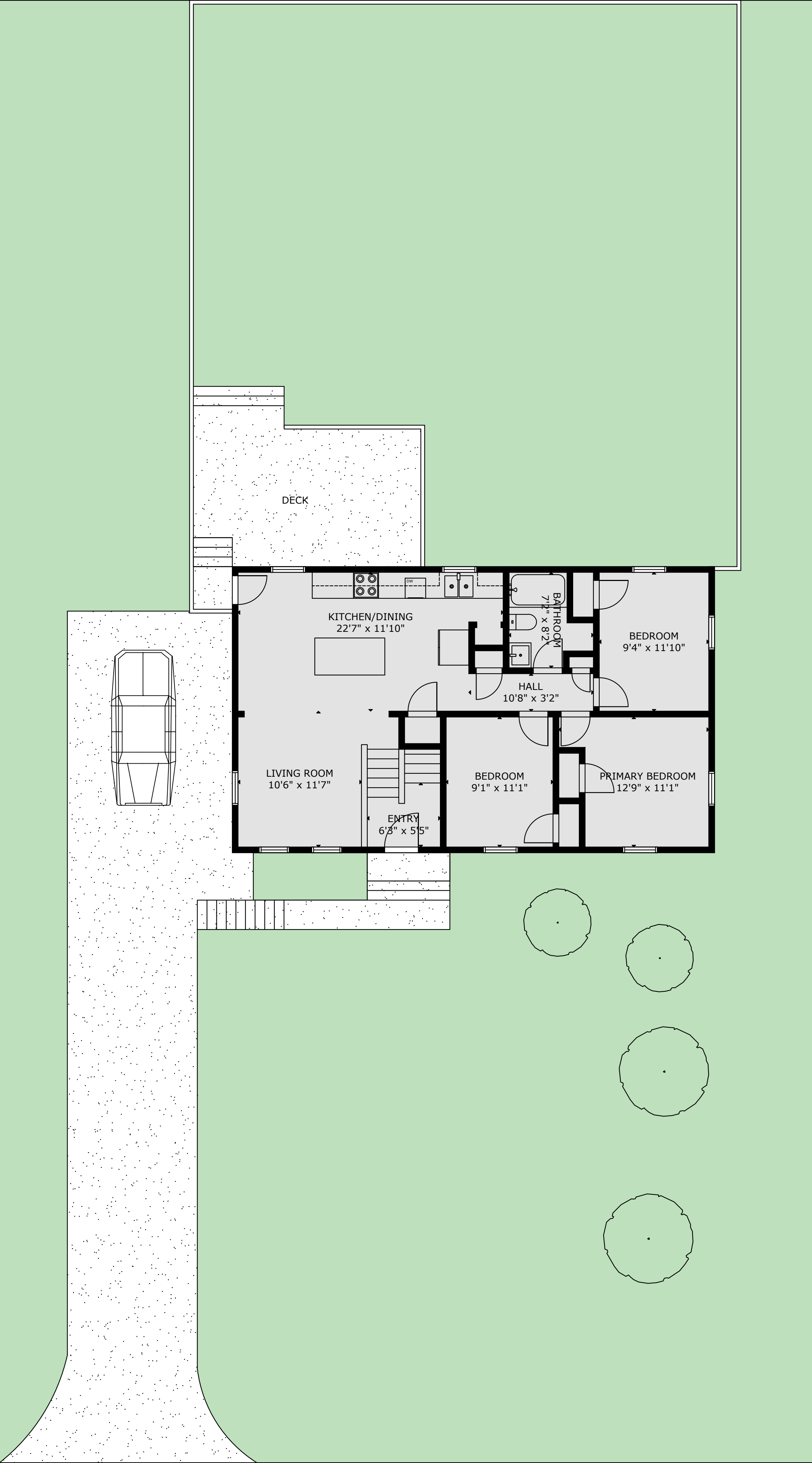
SITEPLAN
