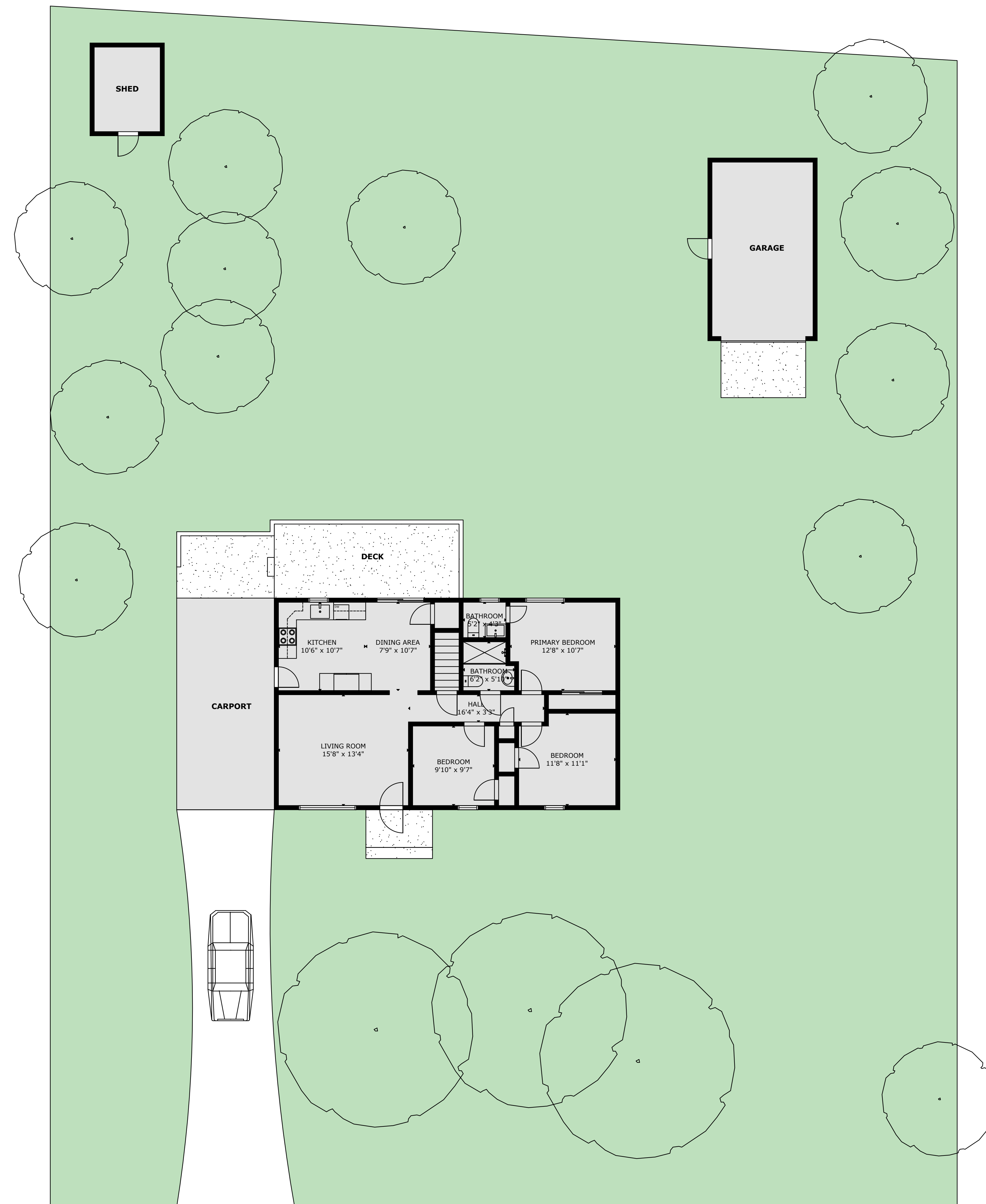
SITEPLAN
