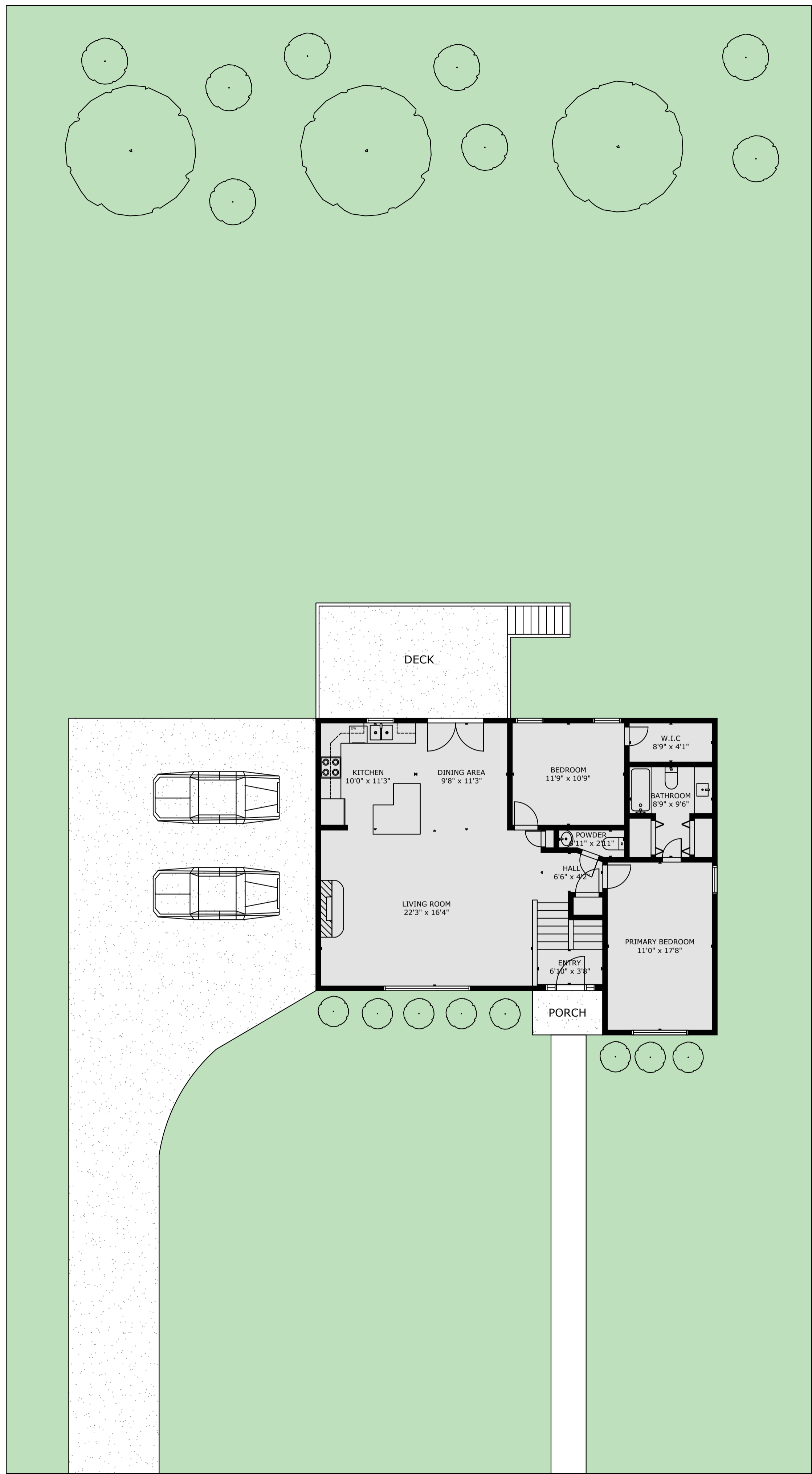
SITEPLAN
