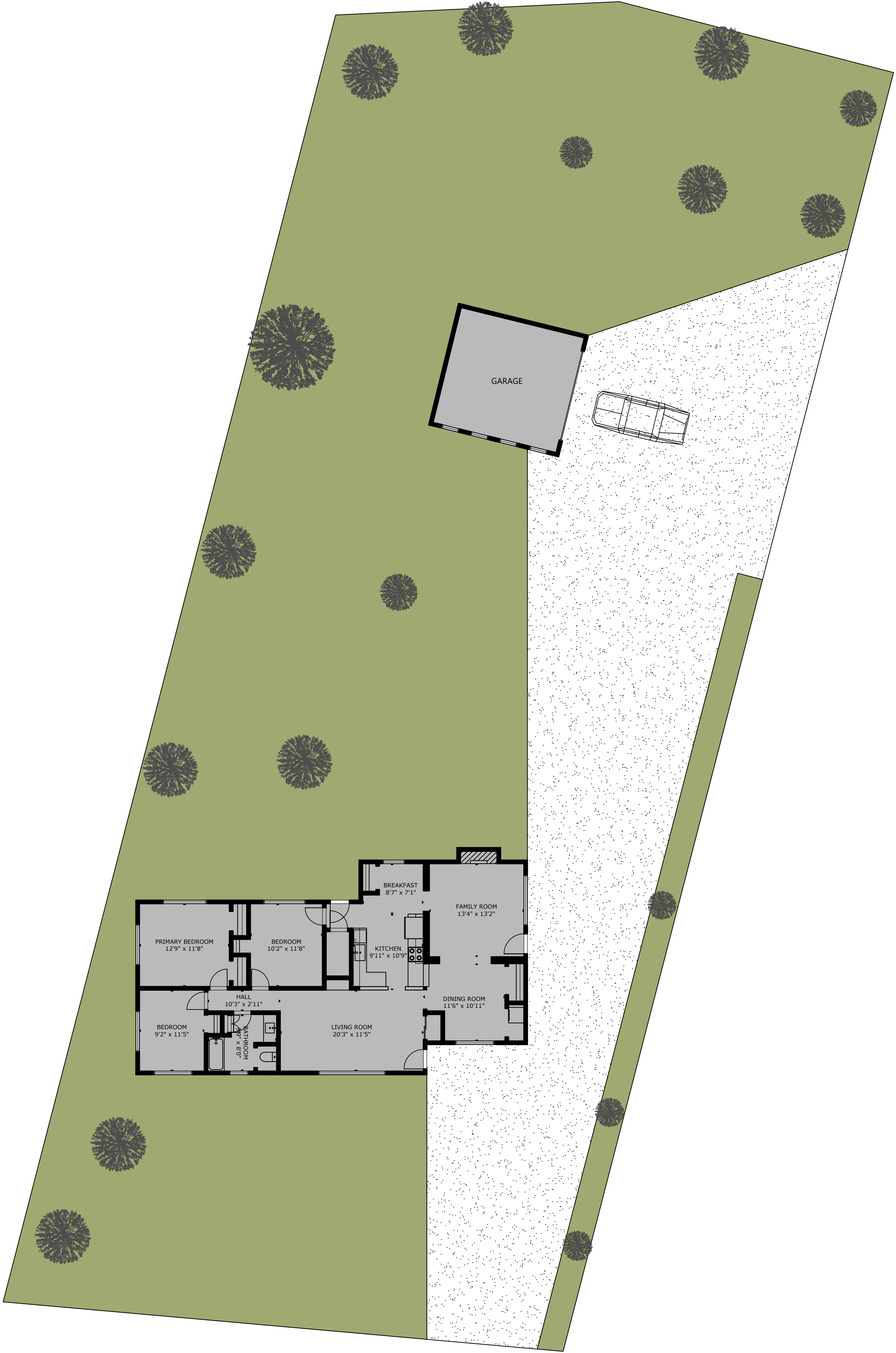
SITEPLAN
