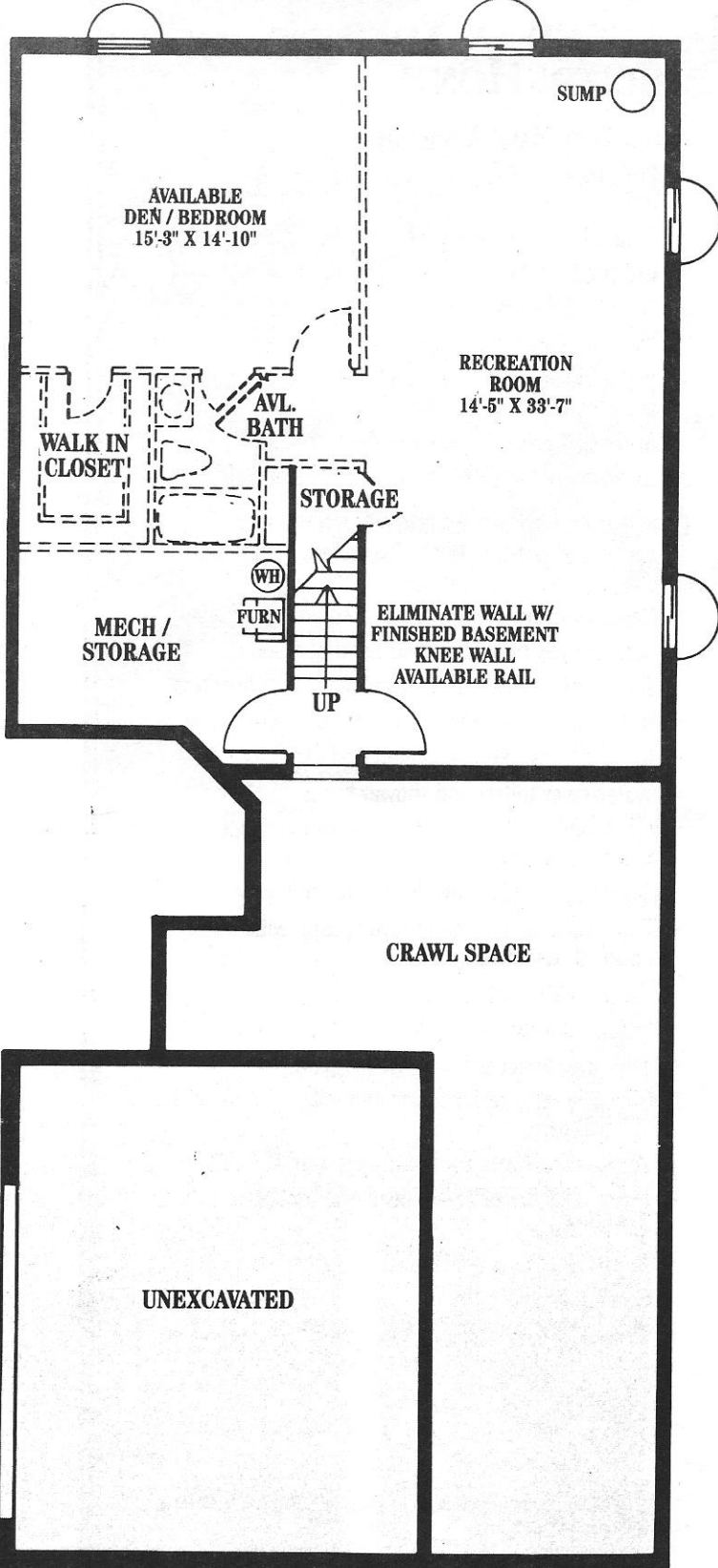
OPTIONAL BASEMENT PLAN
